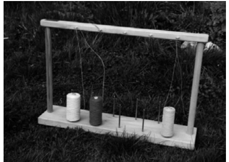
kleiner Schärbaum in 2m und 2.5mUmfang Gewicht: 16 kg
