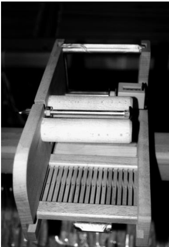
Fadenführgerät mit Zählwerk Einzug- und Auszugwebblatt sowie Gatterkamm zur Fadenkreuzbildung
